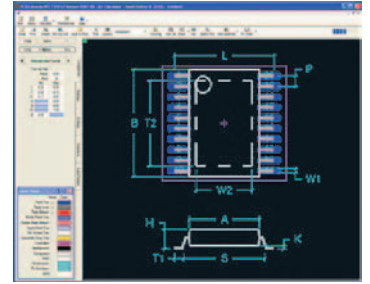
správa součástek
