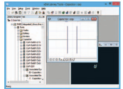
centrální knihovna
